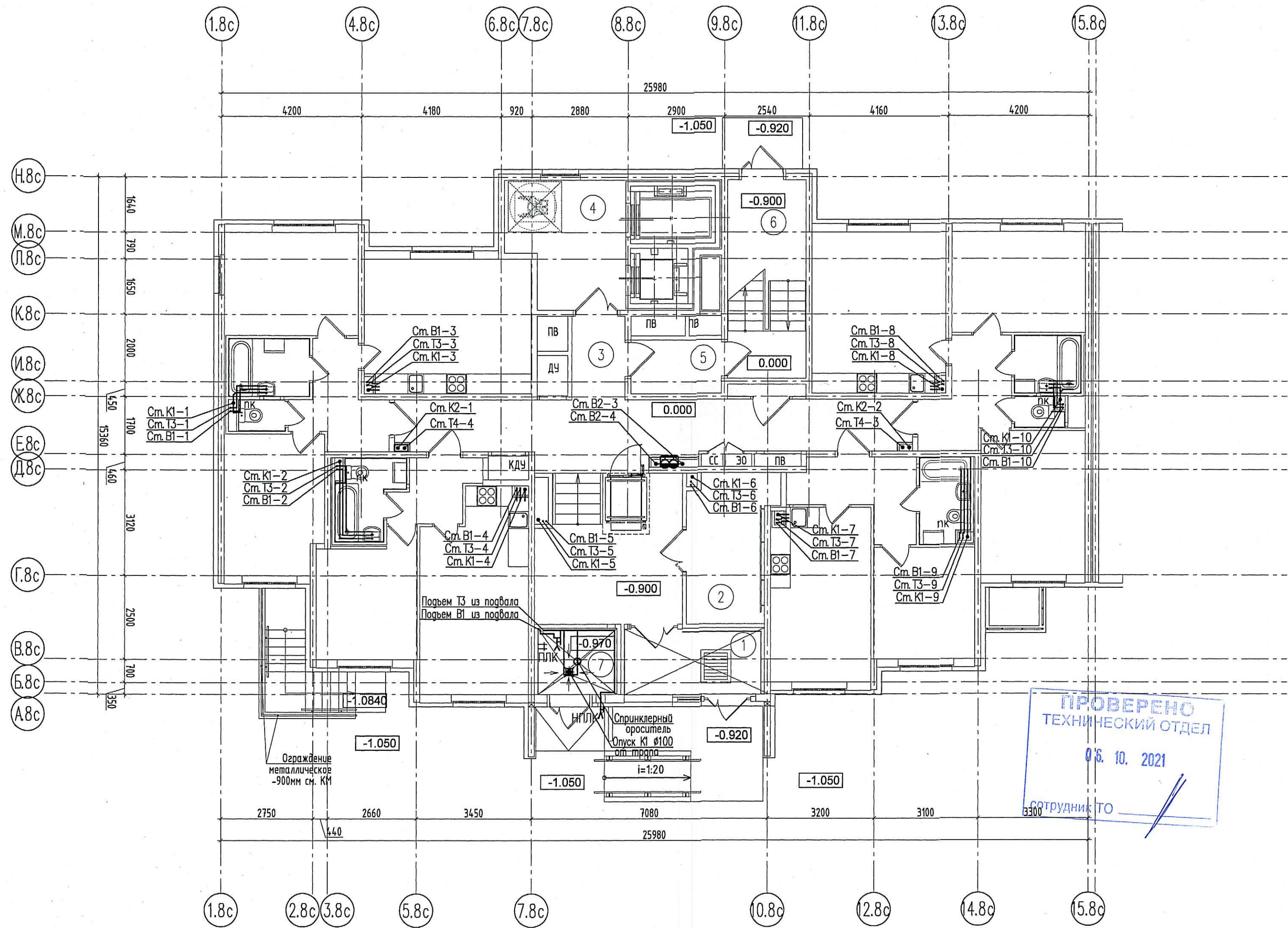
СХЕМА РАСПОЛОЖЕНИЯ СЕКЦИЙ Участок 14
