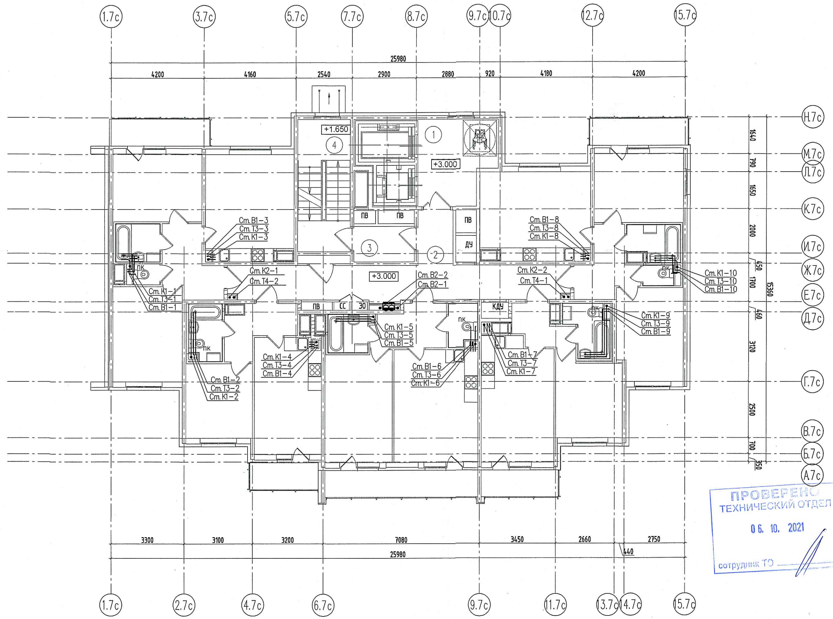
СХЕМА РАСПОЛОЖЕНИЯ СЕКЦИЙ Участок 14
